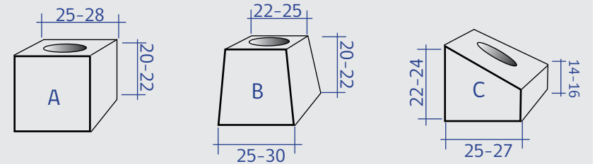
Figura 1: Datos de hormigón.
